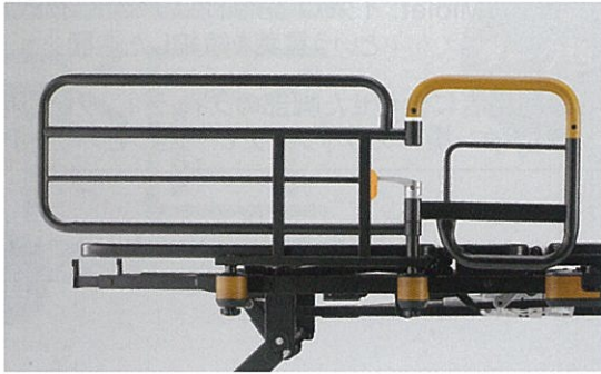
回転式アーム介助バー K-40R TAIS:00167-000138 ※アーム部の角度は15°刻みで調節可能
