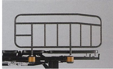
サイドレール K-170S TAIS:00167-000110 ※ショートサイズ足側専用
